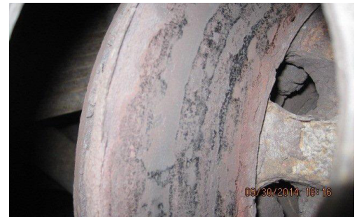
Rusted Rotor. OOSC, Part II, a.(6)(d) or a.(7)(e) / 393.48(a)-U.S.
